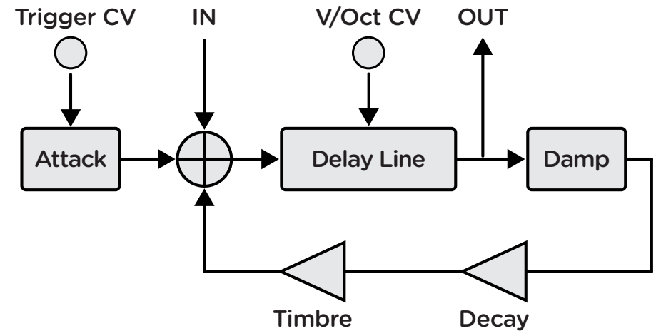
SuperKar+ single voice ブロック図
